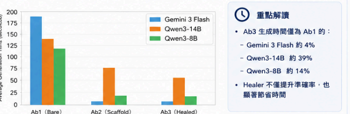
附圖 3：雲端模型與邊緣 AI 模型在分數四則運算的生成時間比較
